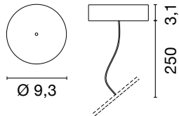
Rosone completo di cavo di alimentazione Ceiling rose with cable
