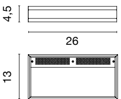
4325 halo 1,1 kg 160W R7s ECO
