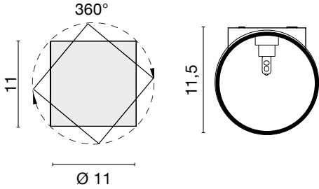
4287 0,5 kg 48W G9 ECO F
