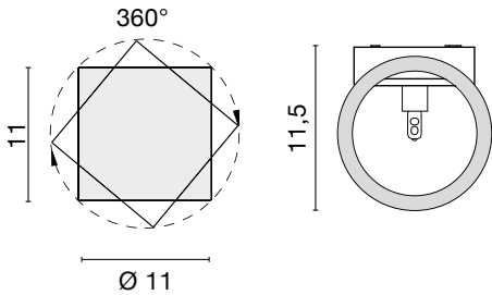
4286 0,5 kg 20-33-48W G9 ECO F
