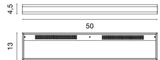
4326 fluo 1,9 kg 36W 2G11
